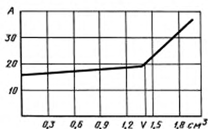
График титрования
